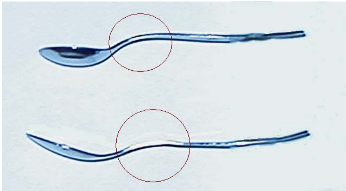
Kuvio 4. Tutkijan työpaikan keittiön alle 5 vuotta tavanomaisessa käytössä olleita kahvilusikoita. Tarkastelussa havaitut taipumakohdat korostettu ympäröimällä. (Kuva: mrkala, Helsinki 24.1.2006)
